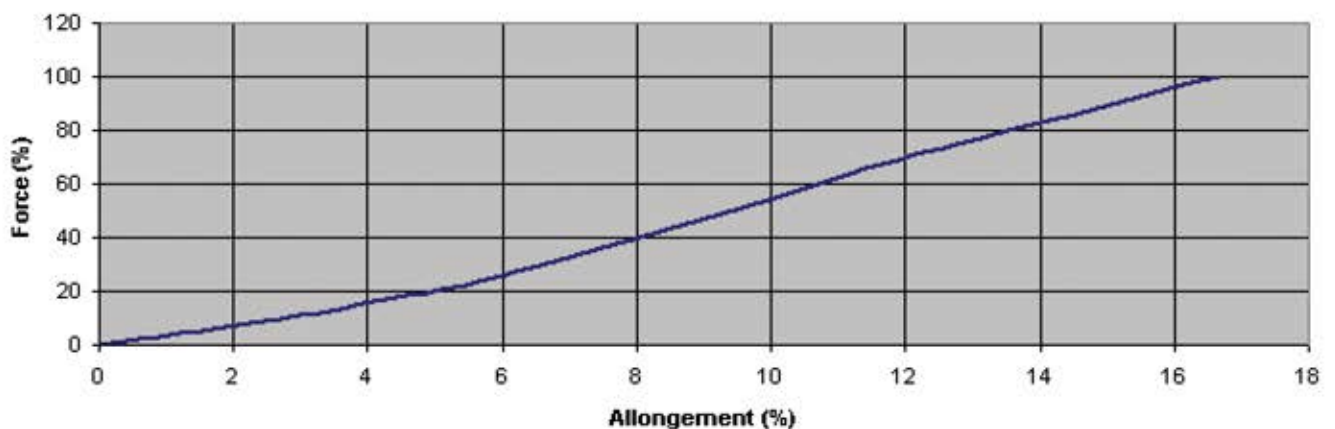
Courbe Force Allongement à la rupture prétension de 1 % *
